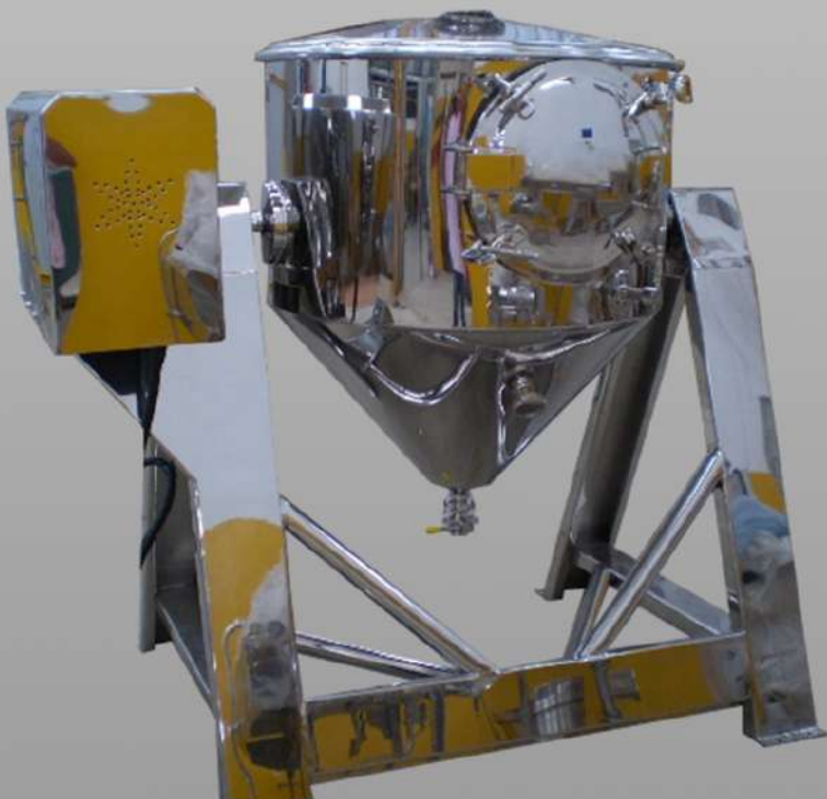
Batedeira Cônica
