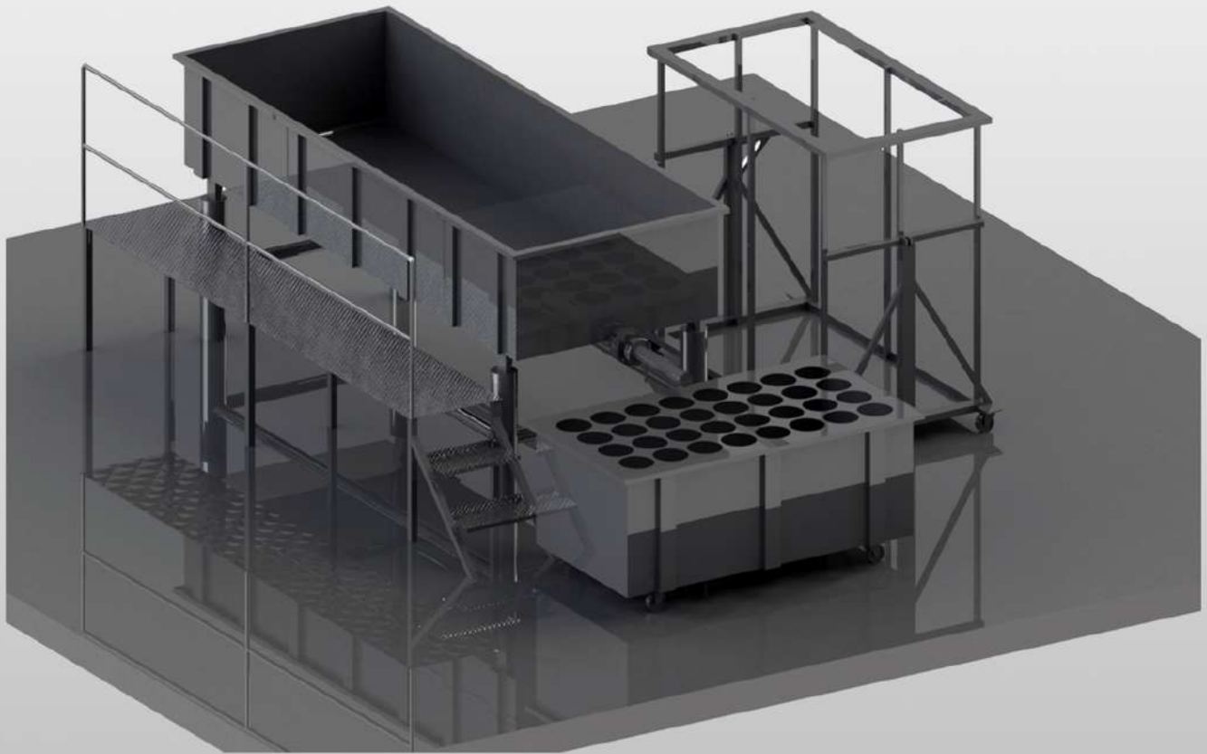
Planta Para fabricação de Frescal, Gorgozola e Ricota
